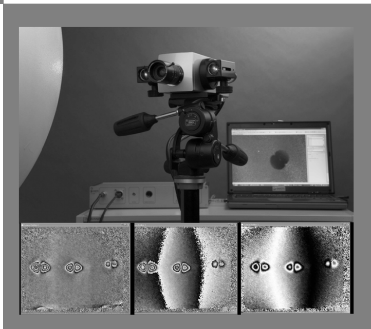
Q-800 シェアログラフィー 非破壊検査システム
